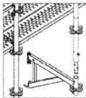
Typ 1 Konsol utan tapp.
