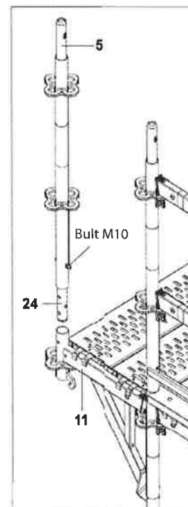
Typ 3 Konsol med svetsad tapp.
